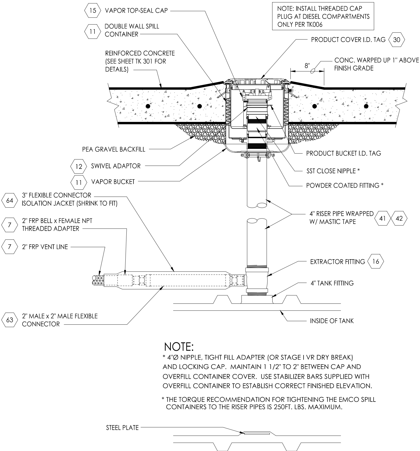
5 VAPOR RISER DETAIL
